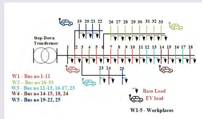
الشكل (2): شبكة توزيع طاقة الموصل العمومي IEEE 33 قيد الدراسة.
