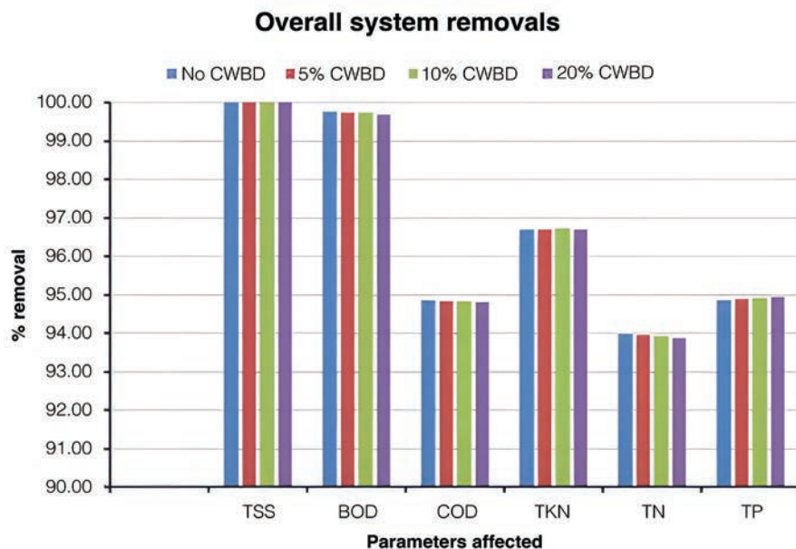
الشكل (2): عمليات الإزالة في المنظومة بشكل شامل بدون المياه الراجعة من محطات تبريد المناطق، وفي حال وجودها بنسبة 5% أو 10% أو 20%.
