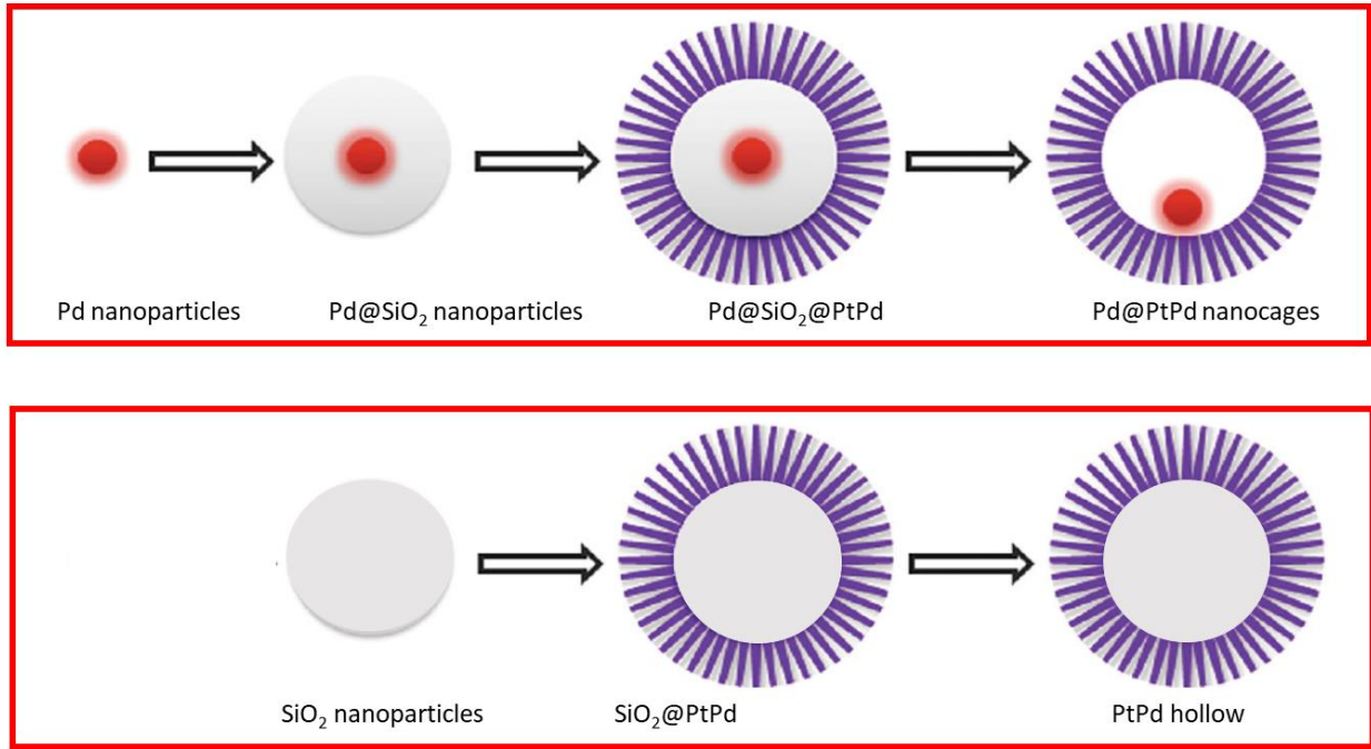
الشكل (1): تصنيع الأقفاص النانوية الجوفاء للمركب المكون من البلاتينوم والبلاتين. (أ) البلاتينوم والبلاتين مع نواة البلاتينوم (Pd*PtPd)، (ب) البلاتينوم والبلاتين (PdPt).
