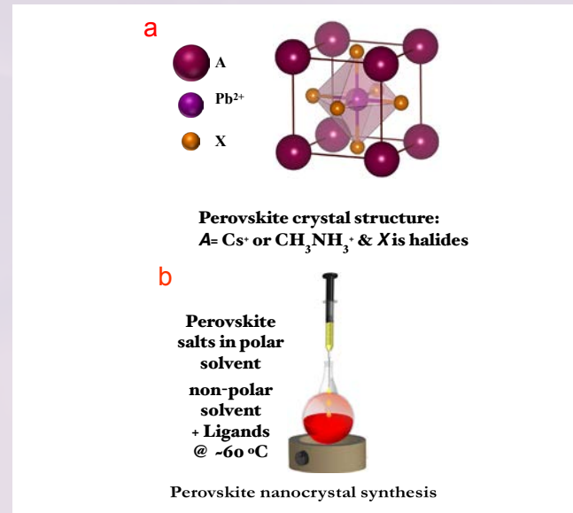
الشكل (1): (a) التركيب البلوري لعائلة بيروفسكايت هاليد الرصاص. (b) مخطط توضيحي لطريقة التحضير المعملية لمواد بيروفسكايت هاليد الرصاص النانومترية باستخدام طريقة إعادة الترسيب بمساعدة الأحماض العضوية.
