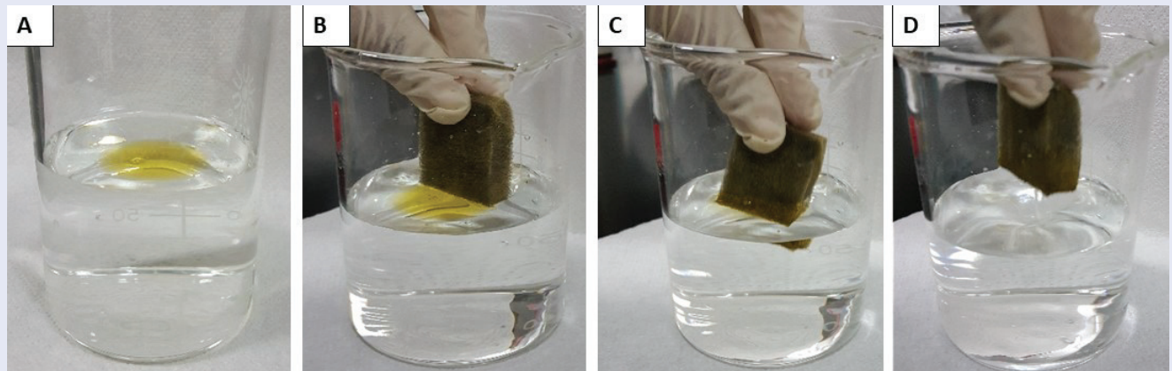
الشكل (2): صور رقمية لامتصاص الانتقائي للزيت في خليط من الماء والزيت باستخدام إسفنجة البولي يوريثين المَطلية بأكسيد الجرافين المُختزل.
