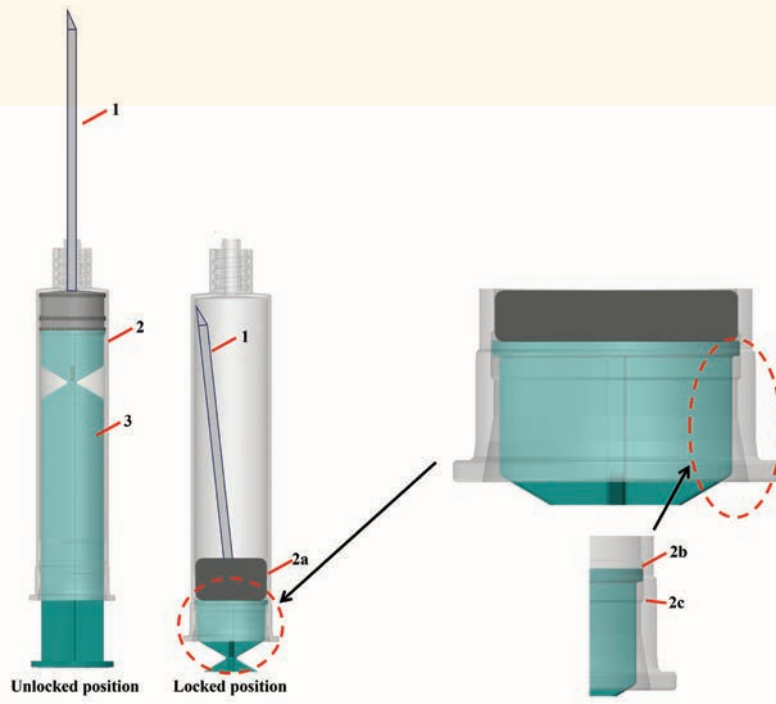
الشكل (2): وصف تصميم المحقنة الآمنة الجديدة.
