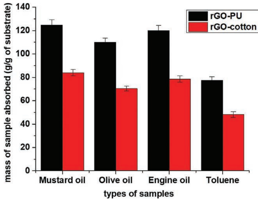
الشكل (4): قدرة امتصاص إسفنجية البولي يوريثين المُطلي بأكسيد الجرافين المُختزل والقطن المُطلي بأكسيد الجرافين المُختزل لمختلف العينات.
