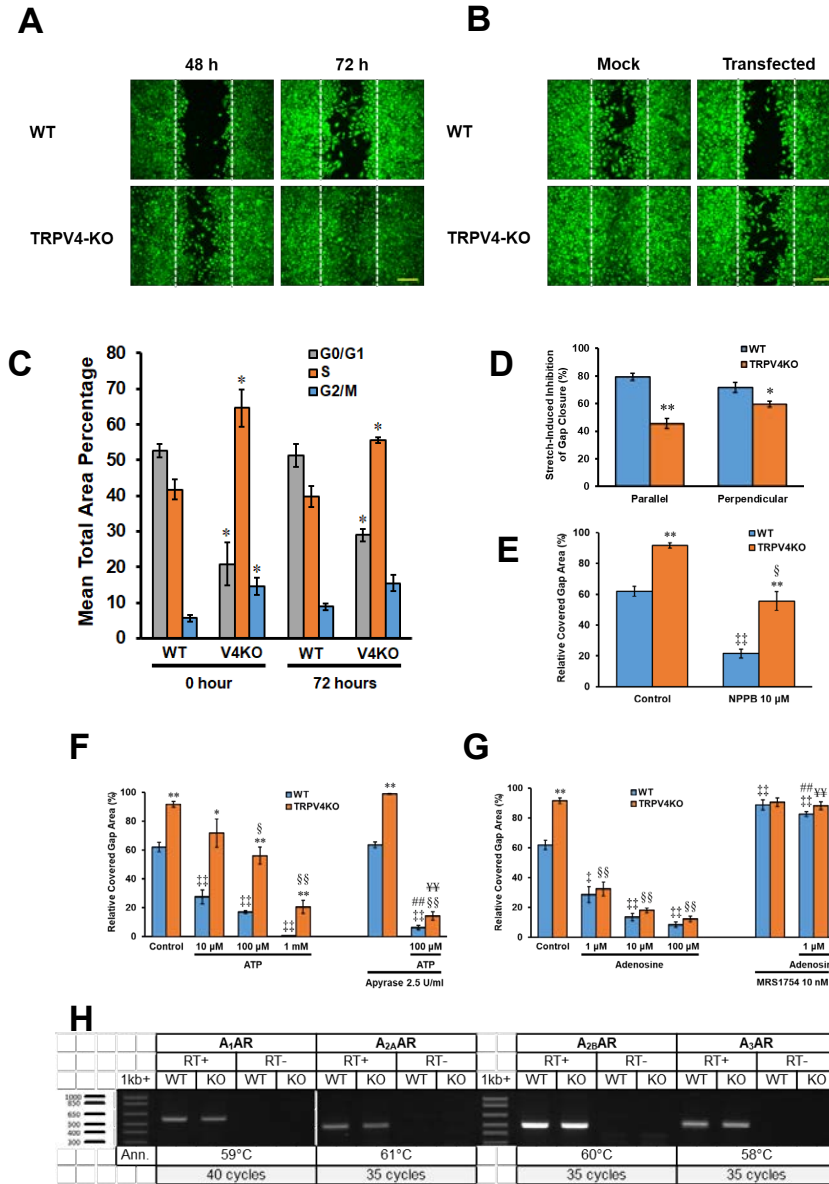
الشكل (1): تنظم قناة TRPV4 عملية التئام جروح الخلايا الكيراتينية المبريتية.
