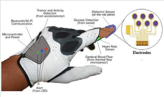
الشكل (7): جهاز استشعار الجلكوز القابل للارتداء.
